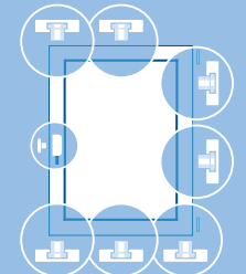
Allseitiger Beschlag mit Achtkantverschlussbolzen + Sicherheitsschließblechen
