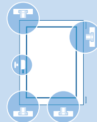
An allen 4 Ecken Achtkantverschlussbolzen + Sicherheitsschließbleche
