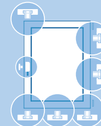
Allseitiger Beschlag mit Achtkantverschlussbolzen + Sicherheitsschließblechen
